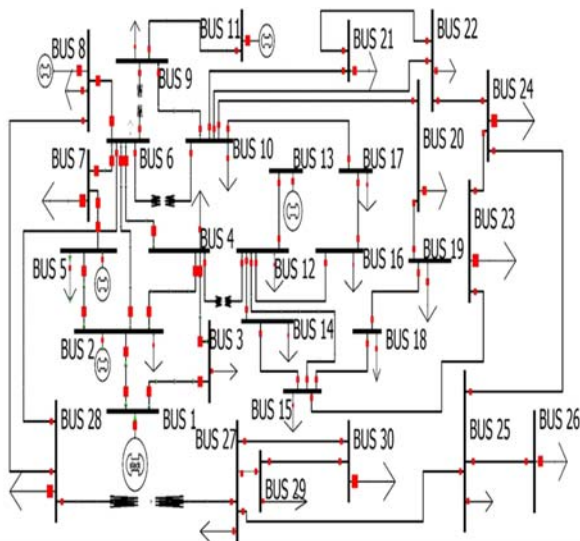
Figure-9. IEEE 30-bus system.
